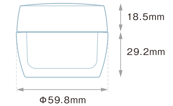
PCI-50 (PP/PP) キャップ (PP) O.F.容量 : 62.4ml
