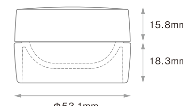
PCL-20 (PP) キャップ (PP)
