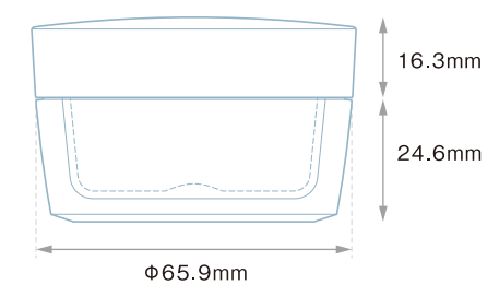
CPA-40 (AS/PP) キャップ (ABS) O.F.容量：56.3ml
