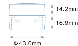
PCL-10 (PP) キャップ (PP)
