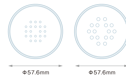
APN パウダー中蓋 (PE)
