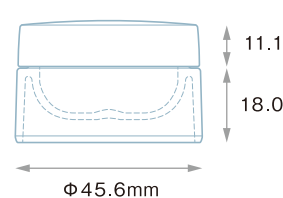
ANC-15 (PP) Fキャップ (PP)
