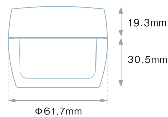
PCI-60 (PP/PP) キャップ (PP) O.F.容量 : 73.3ml
