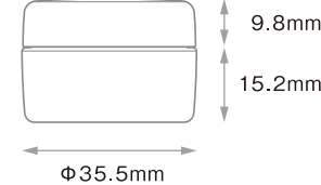
PCN-10 (PP) Rキャップ (PP)
